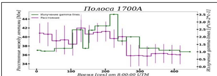
Рис. Сравнение эволюции расстояния между вспышечными лентами в полосе 1700 Å с временным профилем гамма-излучения
