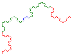
Рис. 2. Кривая Фибоначчи для n = 19 и угла 60
