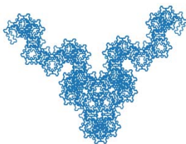
Рис. 3. Кривая Фибоначчи с морфизмом
