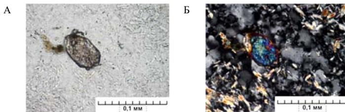
Рис. 2. Микрофотографии циркона в березите: А – при одном поляризаторе, Б – при скрещенных поляризаторах
