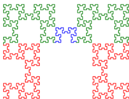
Рис. 1. Кривая Фибоначчи для n = 1
