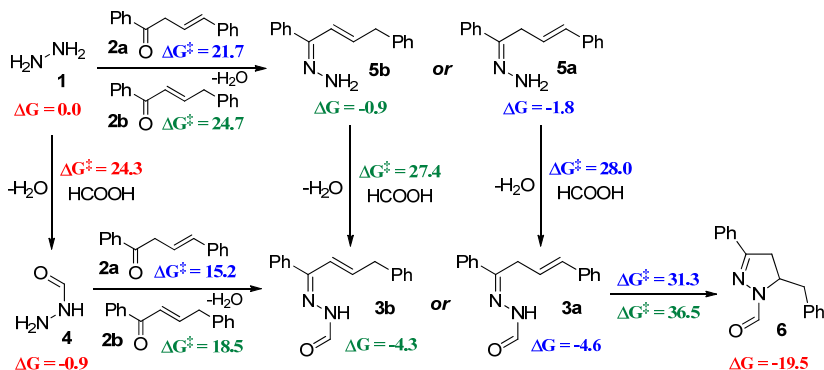
Рис. Сборка 1-формил-2-пиразолина 6 . Значения \Delta G и \Delta G^\ddagger в ккал/моль
